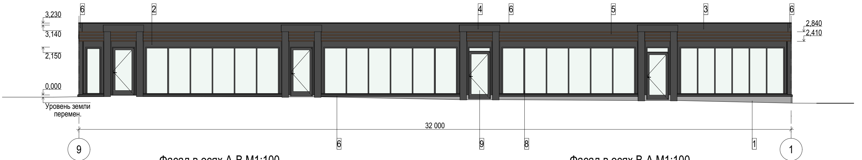
Фасад в осях А-В М1:100
