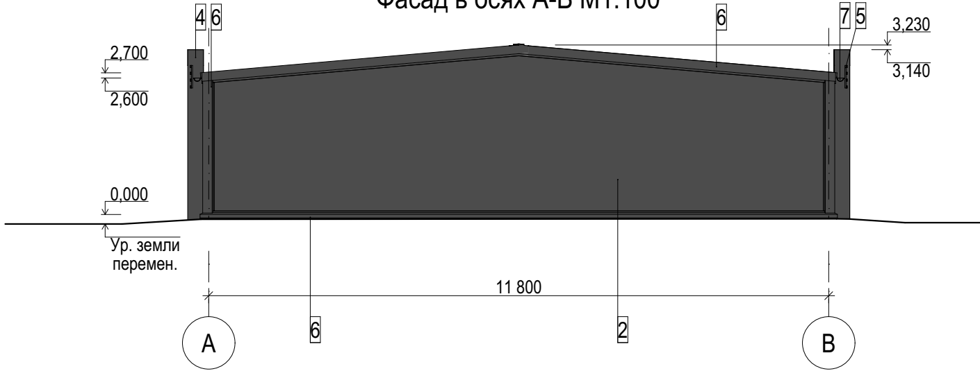
Фасад в осях А-В М1:100
