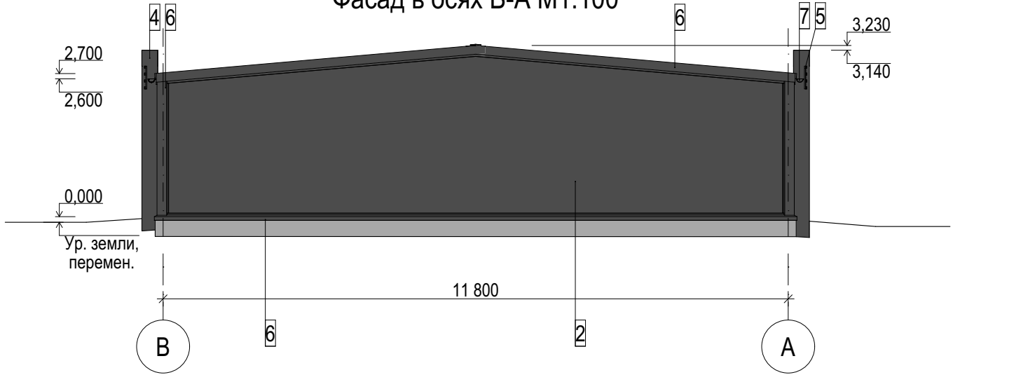
Фасад в осях В-А М1:100
