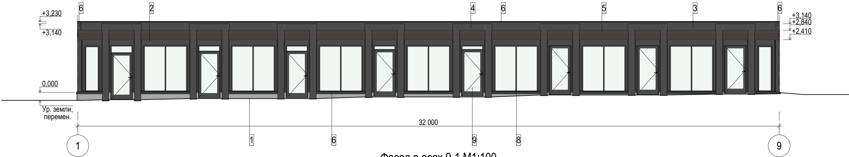
Фасад в осях 9-1 М1:100
